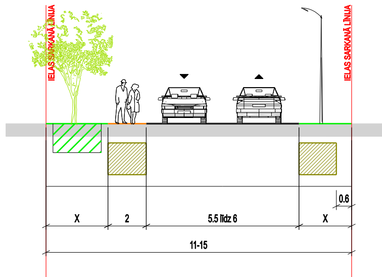
D KATEGORIJAS 5.5 LĪDZ 6 METRUS PLATO BRAUKTUVJU TEORĒTISKAIS GRIEZUMS
