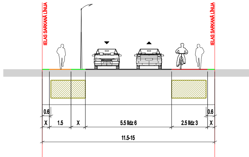
D KATEGORIJAS 5.5 LĪDZ 6 METRUS PLATO BRAUKTUVJU TEORĒTISKAIS GRIEZUMS
