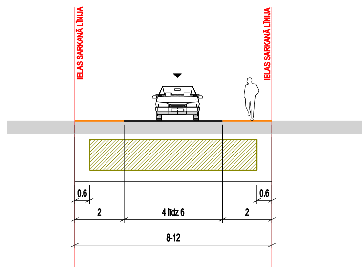
D KATEGORIJAS 4 LĪDZ 6 METRUS PLATO BRAUKTUVJU TEORĒTISKAIS GRIEZUMS
